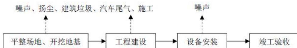
图2-5 施工阶段工艺流程及产污示意图
