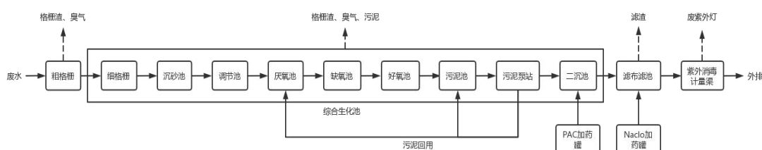
图2-6 项目运营期工艺流程及产污环节图
