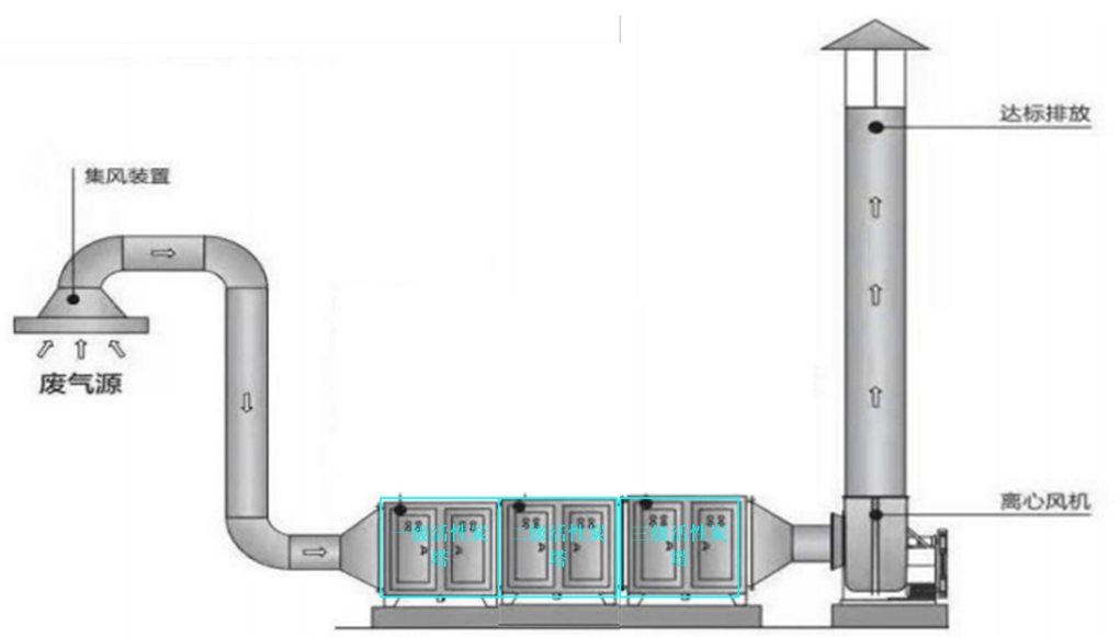
图 4-4 废气治理措施示意图
