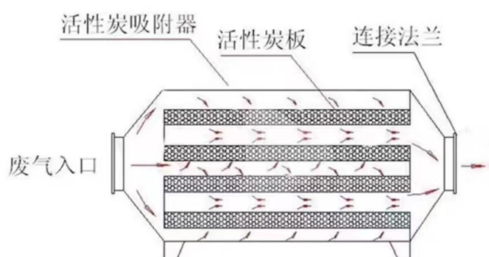
图 4-3 单级活性炭箱内部结构示意图
