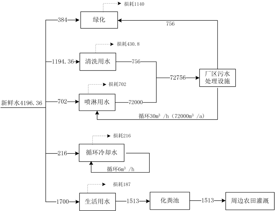
图 2-1 扩建项目水平衡图 (单位: t/a)
