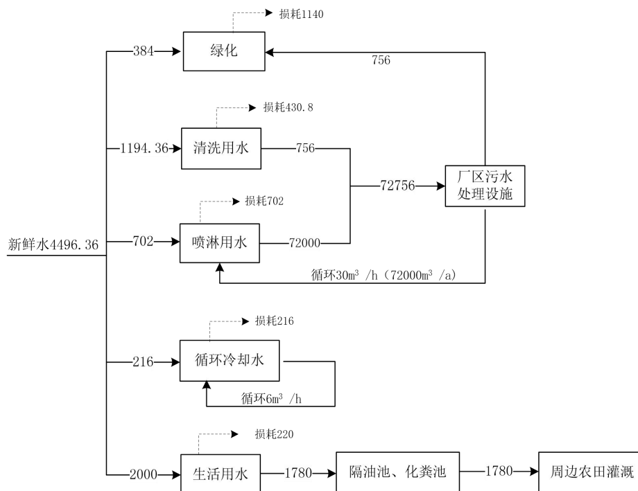
图 2-2 扩建后总水平衡图 (单位: t/a)
