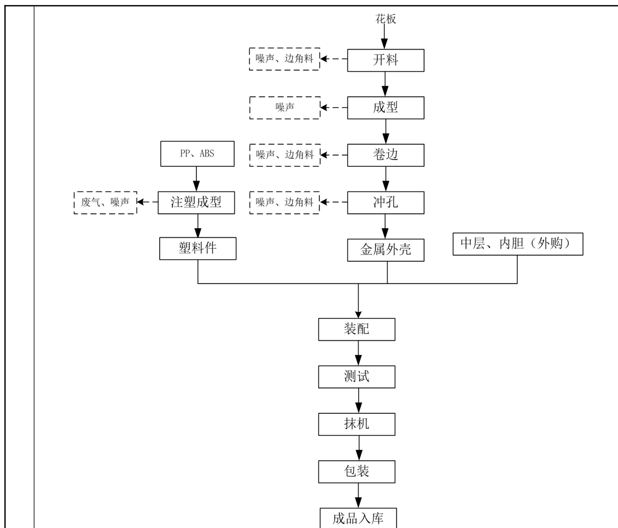
图 2-3 营运期电饭锅工艺流程及产污示意图
