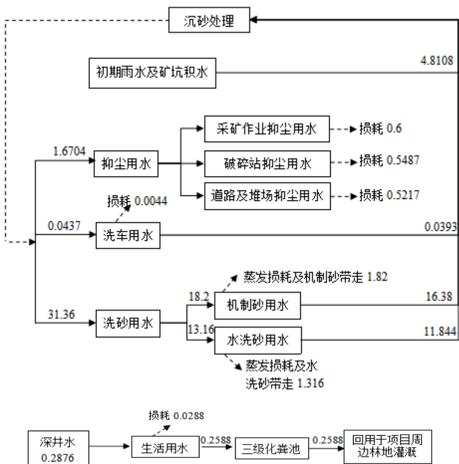
图 2-3 水平衡图 (万 m 3 /a)
