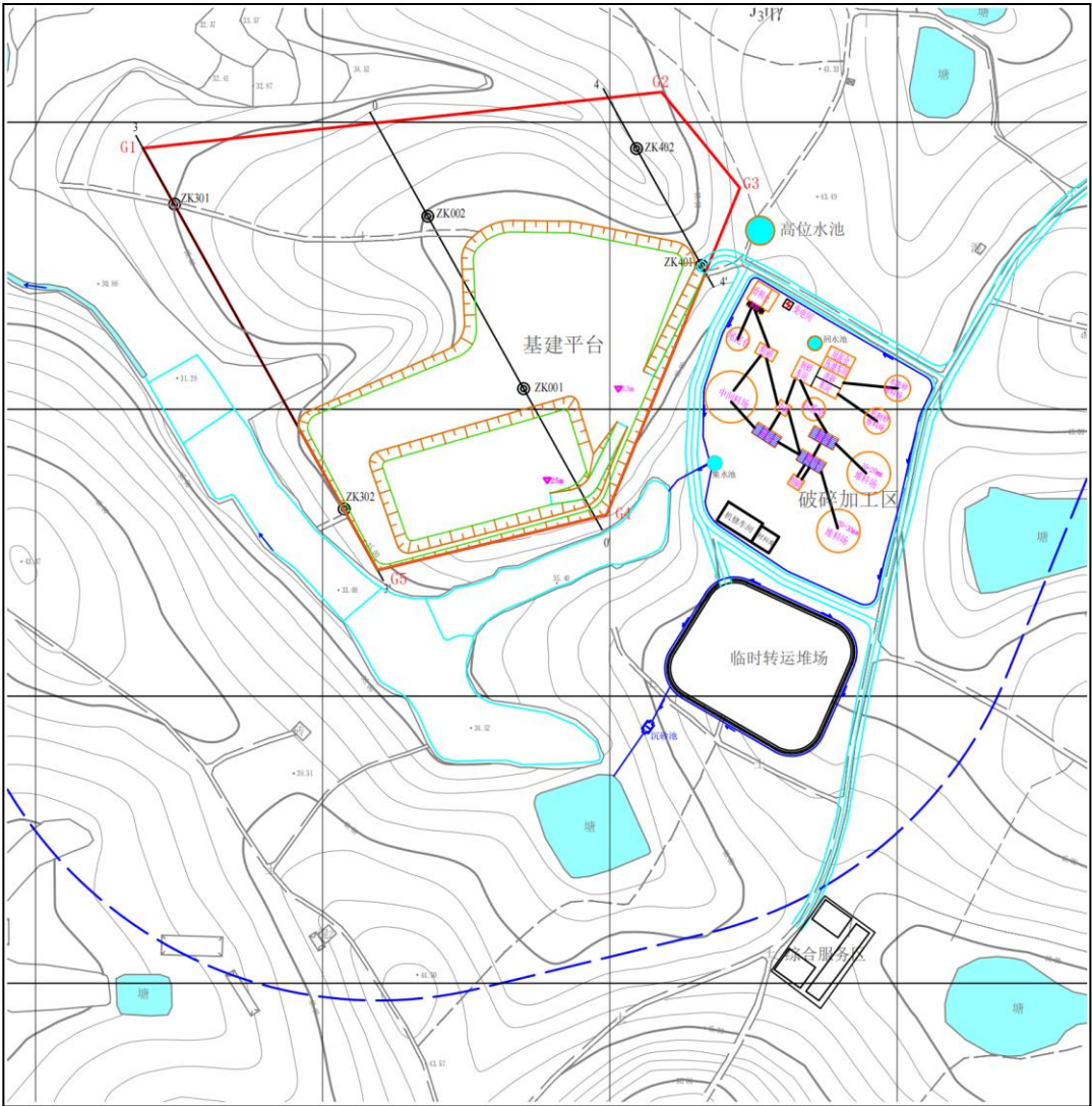
图 2-4.1 本项目工程总布置图
