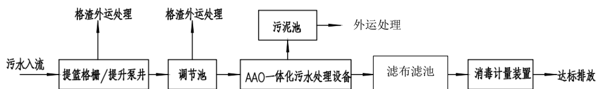
图 2.3 高桥镇(西)水质净化厂污水处理工艺流程图
