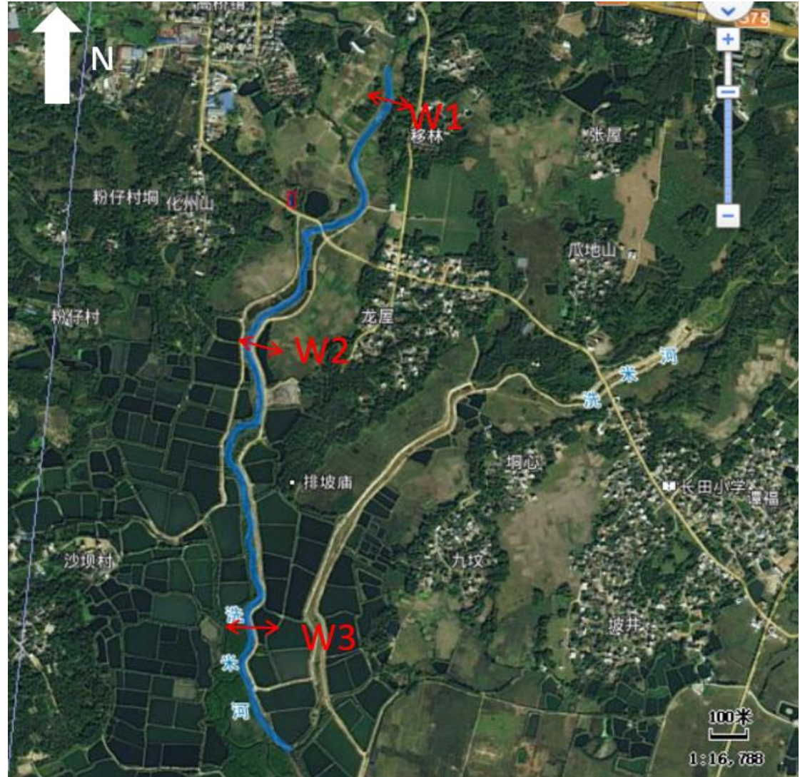
图 3.1 监测断面图
