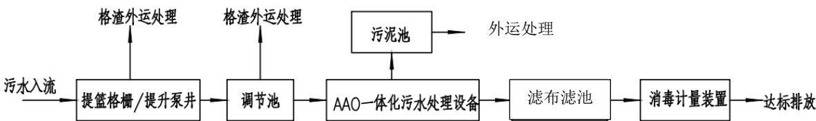
图 2-1 高桥镇（西）水质净化厂污水处理工艺流程图
