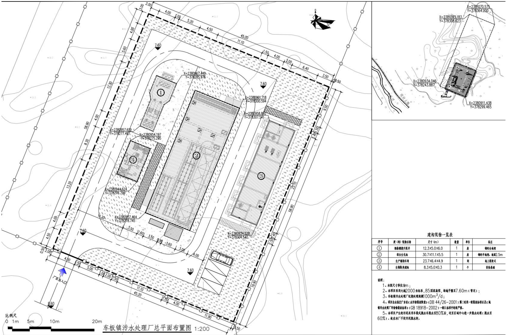
附图4 总平面布置图
