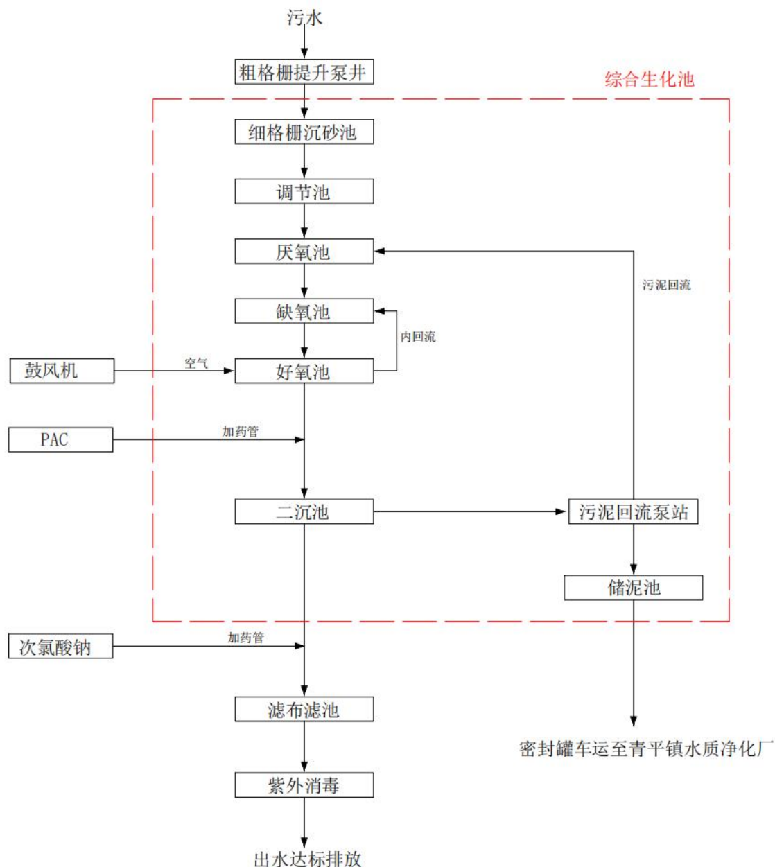
图2-2 车板镇水质净化厂污水处理工艺流程图
