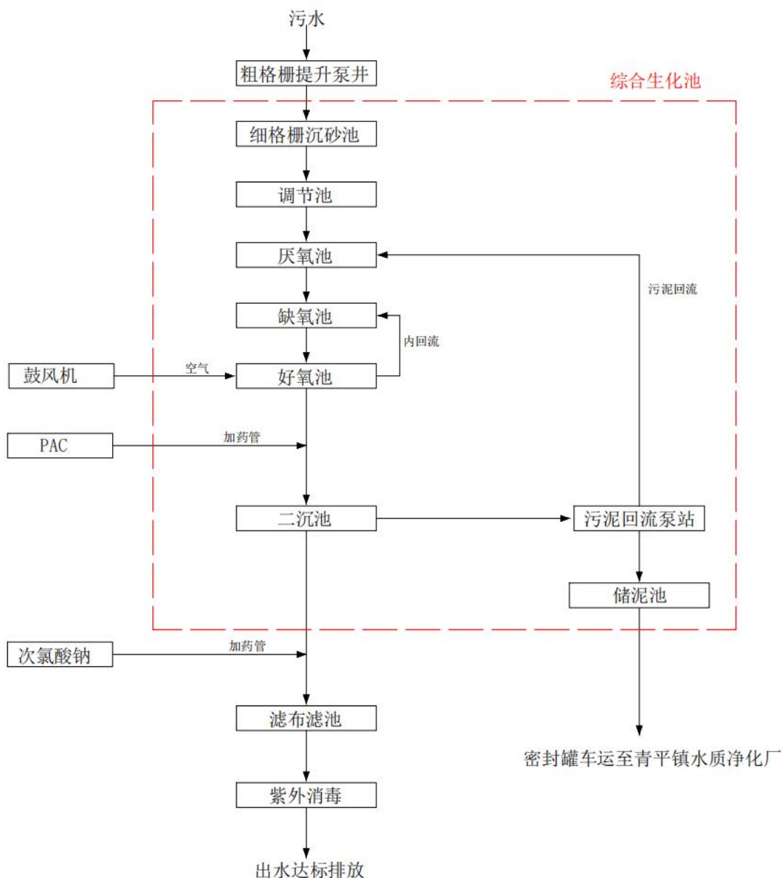
图2.3 车板镇水质净化厂污水处理工艺流程图
