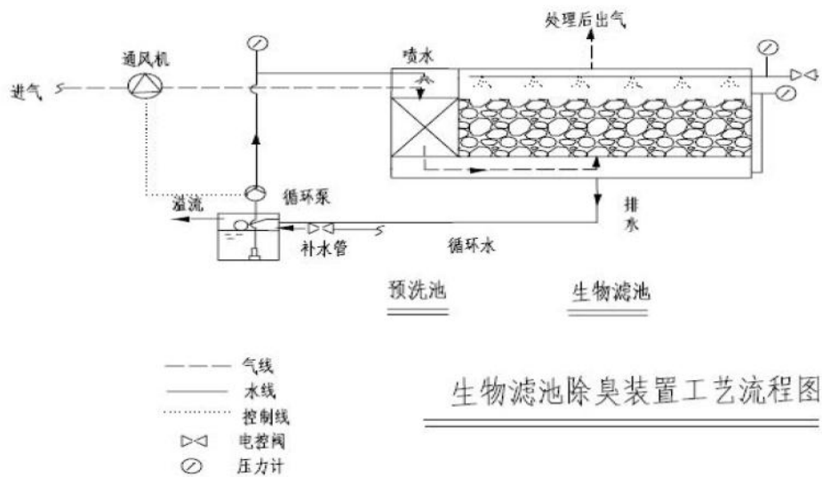
图4-1 生物滤池脱臭工艺流程图
